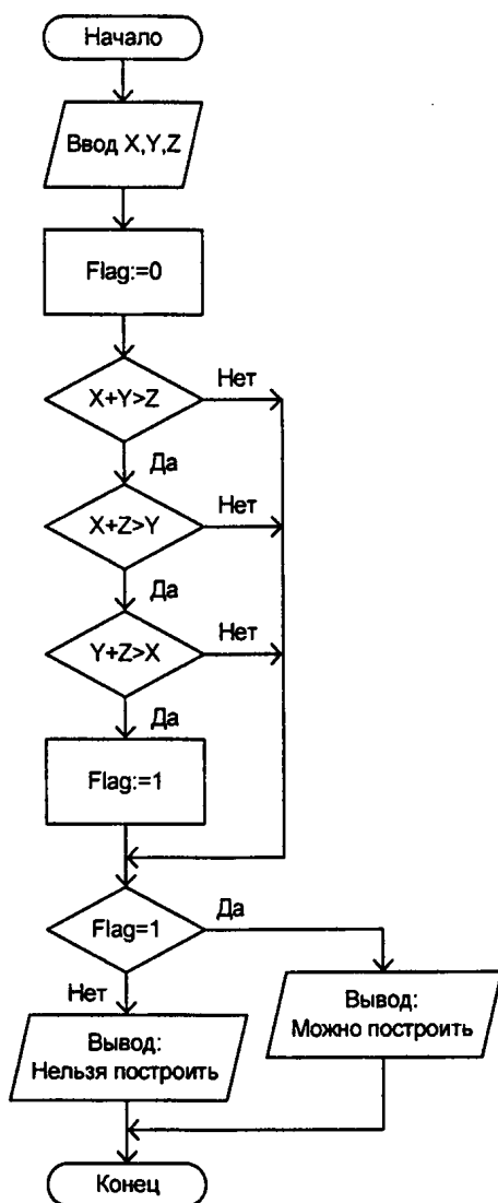
Рис. 2.16. Блок-схема к программе листинга 2.25
