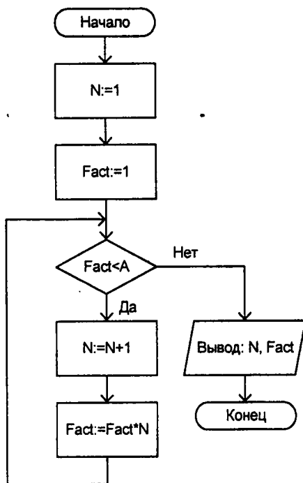
Рис. 2.12. Блок-схема к программе листинга 2.16
