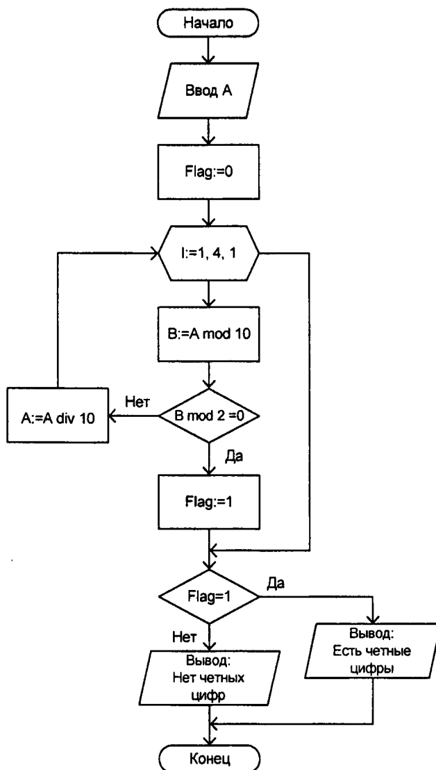
Рис. 2.19. Блок-схема к программе листинга 2.34
