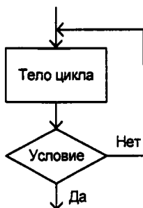
Рис. 2.13. Блок-схема с постусловием
