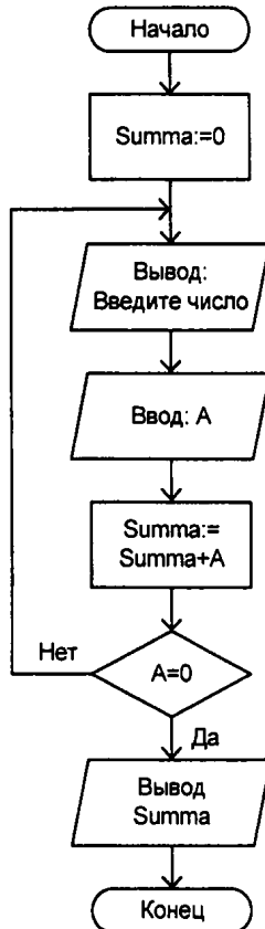
Рис. 2.14. Блок-схема к программе листинга 2.17
