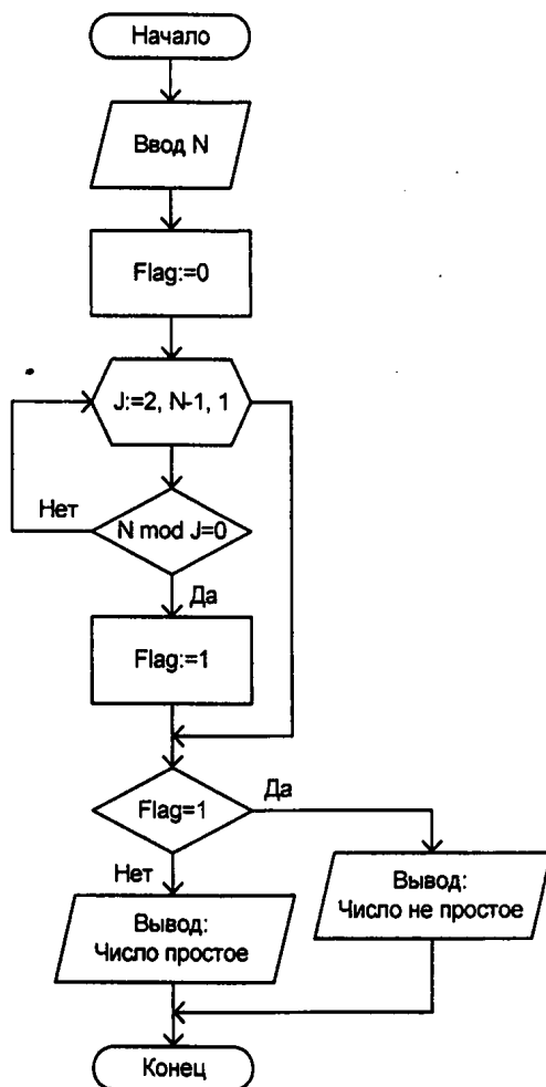
Рис. 2.9. Блок-схема к программе листинга 2.14
