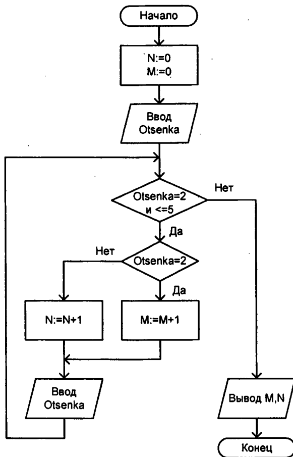
Рис. 2.17. Блок-схема к программе листинга 2.28
