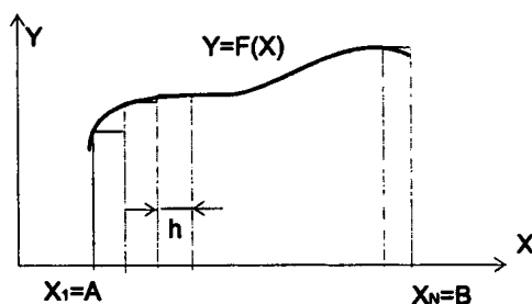
Рис. 8.2. График функции формулы 8.2 с разбивкой на прямоугольники
