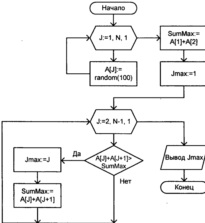
Рис. 3.6. Блок-схема к программе листинга 3.9
